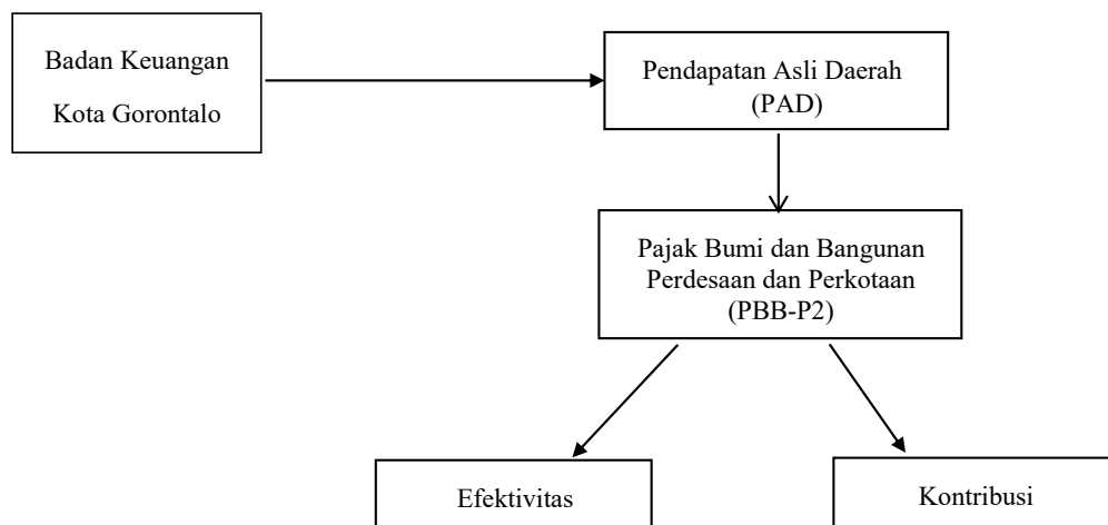
Gambar 1 Kerangka Pemikiran
