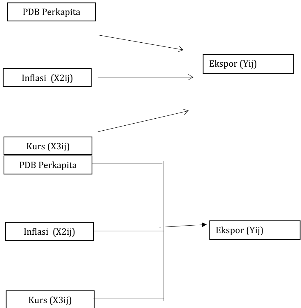
Gambar 1. Kerangka Berpikir
