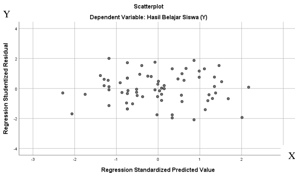
Gambar 1. Scatterplot (Uji Heteroskedasditas)
